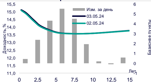
Кривая ОФЗ
